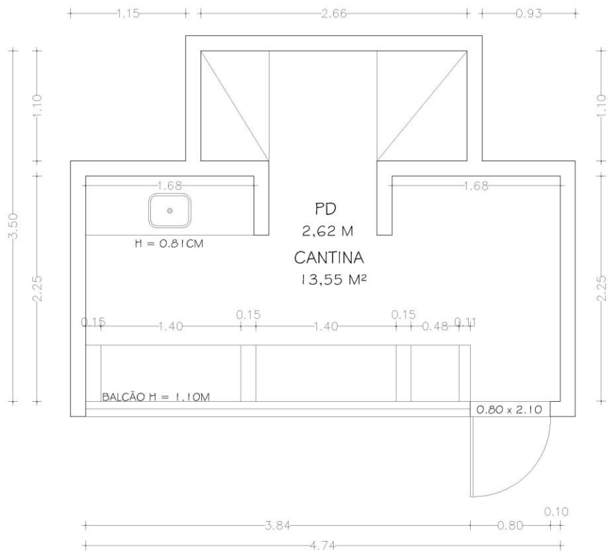
Figura 4-23 - Planta Baixa – Espaço Cantina
