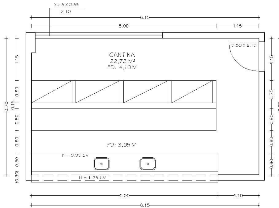
Figura 4-13 - Planta Baixa – Espaço Cantina
