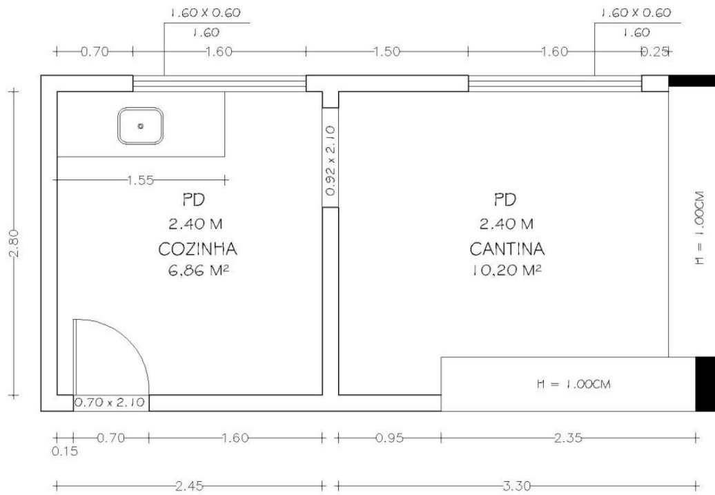
Figura 4-25 - Planta Baixa – Espaço Cantina
