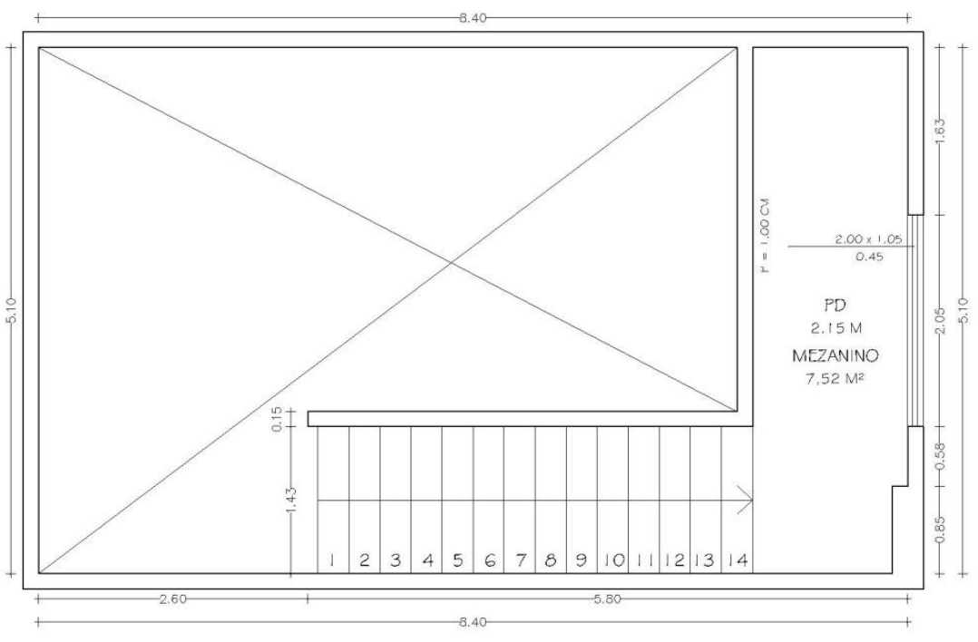
Figura 4-21 - Planta Baixa – Espaço Reprografia
