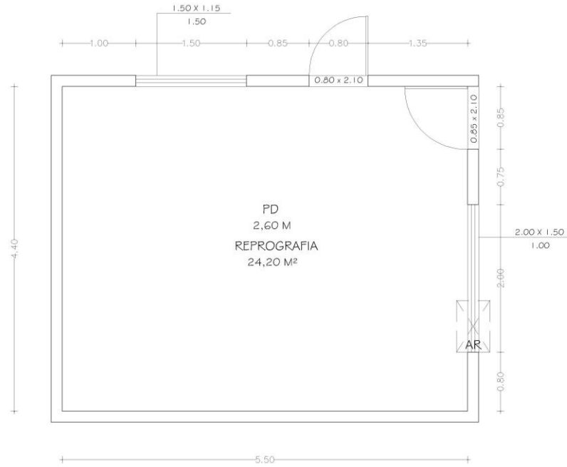
Figura 4-35 - Planta Baixa – Espaço Reprografia
