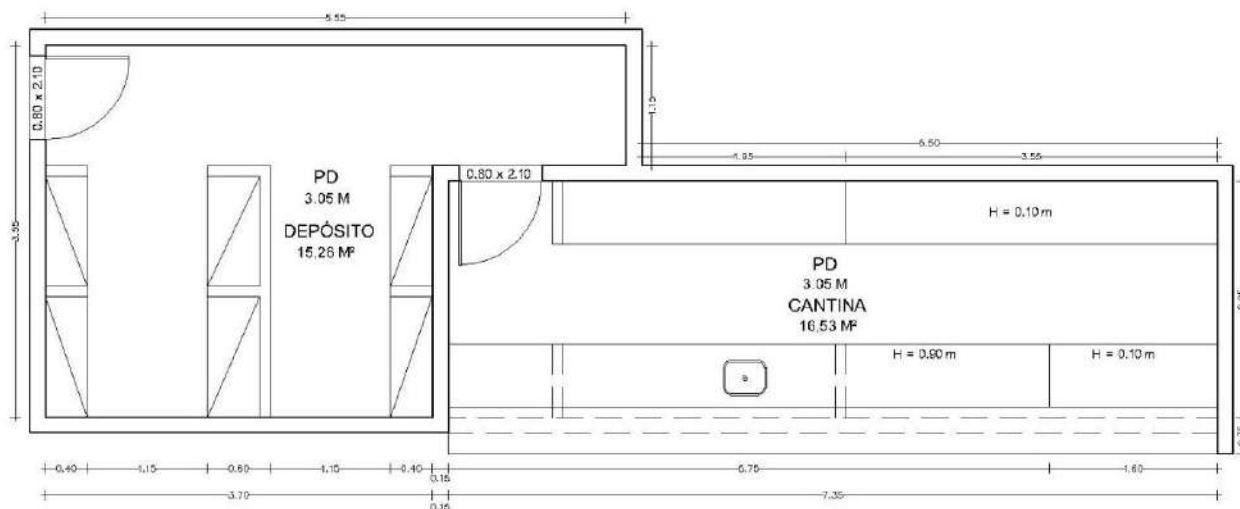
Figura 4-11 - Planta Baixa – Espaço Cantina
