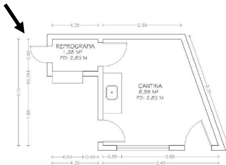
Figura 4-16 - Planta Baixa – Espaço Reprografia
