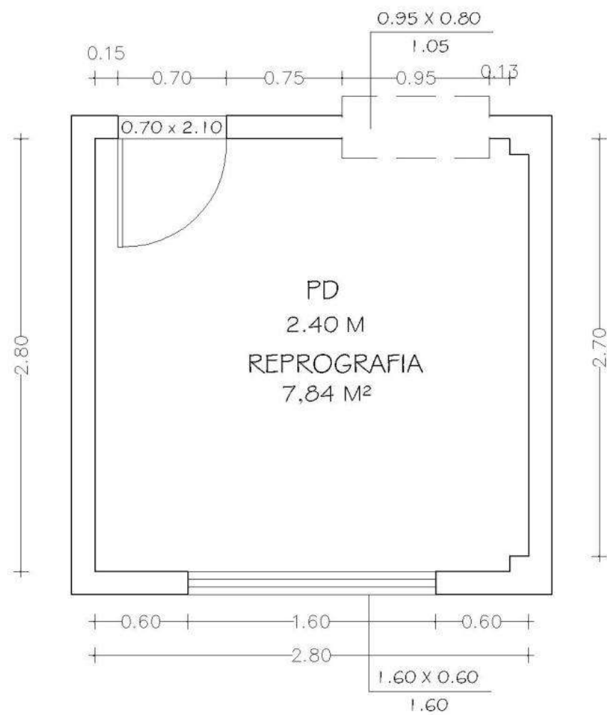
Figura 4-26 - Planta Baixa – Espaço Reprografia
