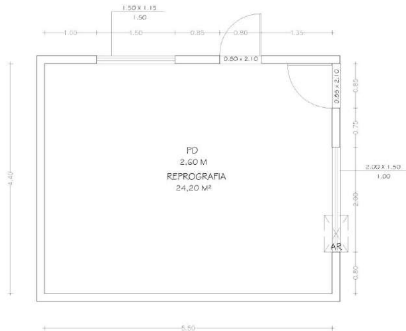
Figura 4-35 - Planta Baixa – Espaço Reprografia
