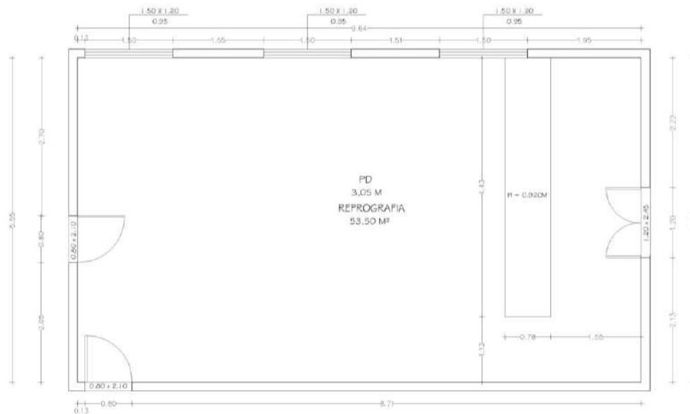
Figura 4-37 - Planta Baixa – Espaço Reprografia
